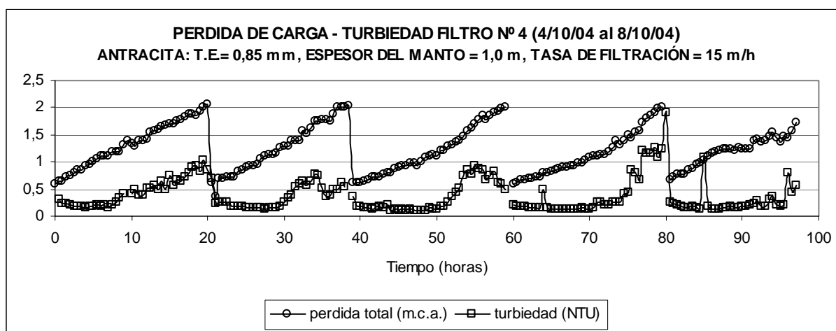
Gráfico N°1: Evolución de pérdidas de carga y turbiedades en un filtro piloto durante una campaña de trabajo
