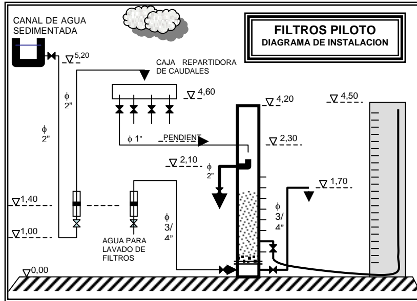
Figura 1: Diagrama de la Planta de Filtros Piloto
