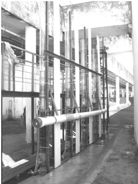
Imagen 1: Vista General de la Planta Piloto
